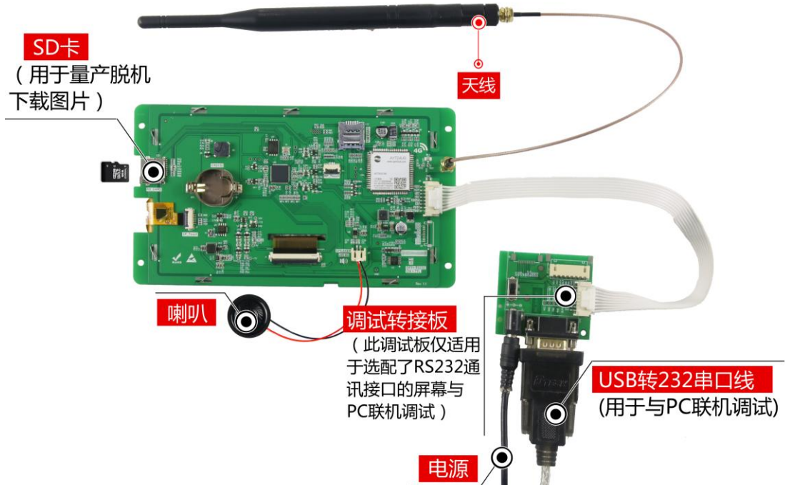
图 1-5 调试工具图
