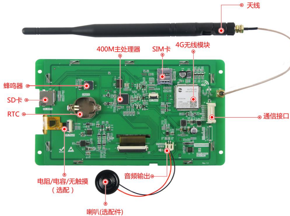
图 1-4 硬件配置图
